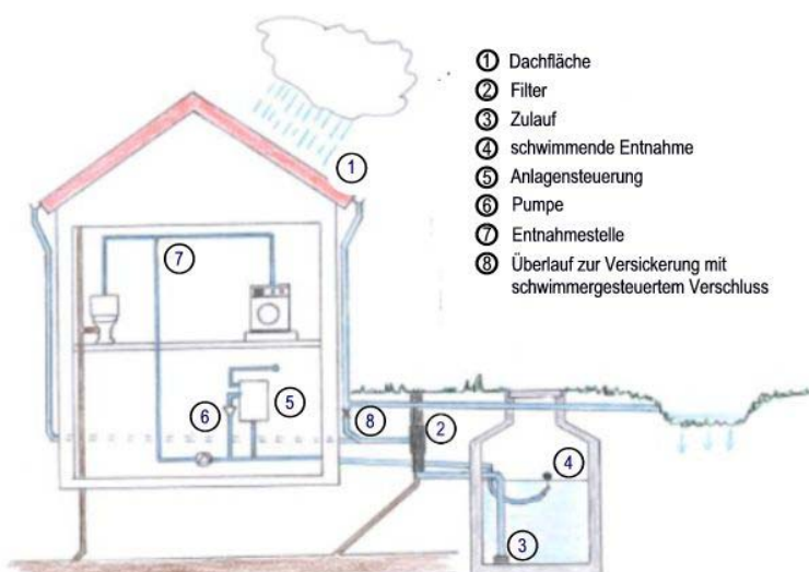
Abb. 16: Regenwassernutzungsanlage (Erdspeicher)
