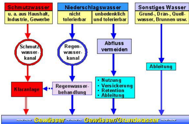
Abb. 5: Modifiziertes Trennsystem (Schemaskizze)
